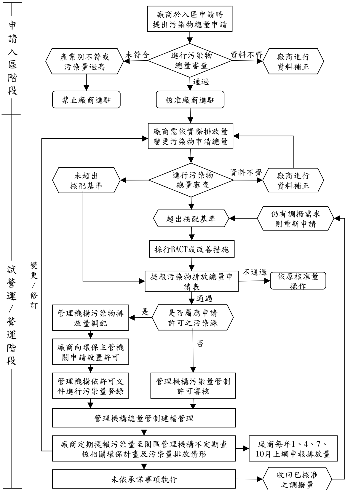
圖 1 南科液晶電視及產業支援工業區(樹谷園區)污染物總量管制審查流程圖
