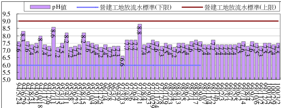
工區放流口放流水質監測結果比較圖(pH值)
