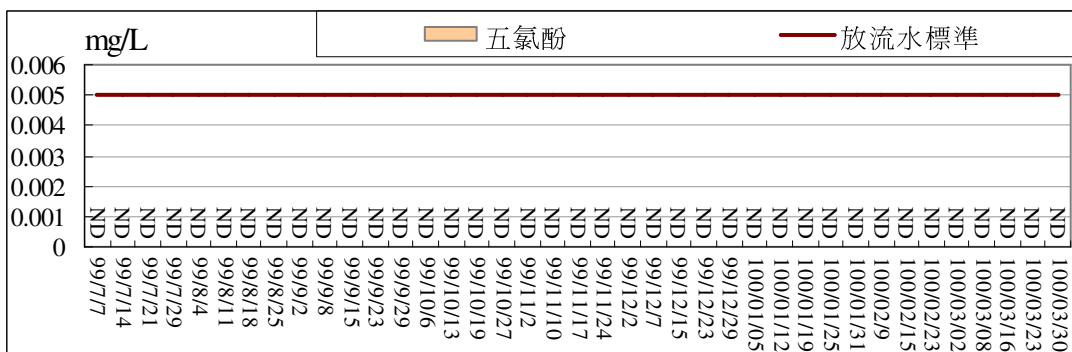
污水處理廠放流口放流水質監測結果比較圖(五氯酚)
