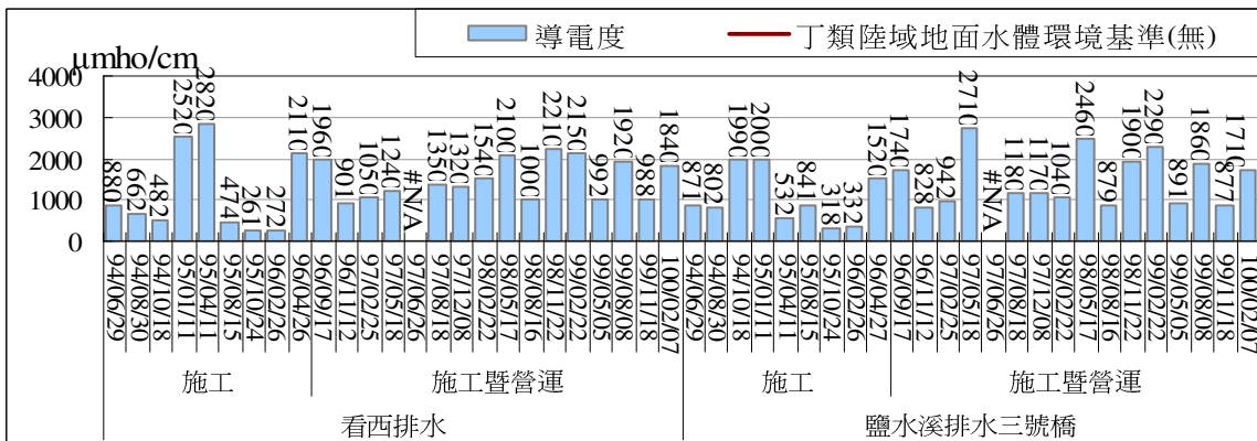
地面水質監測結果比較圖(導電度)
