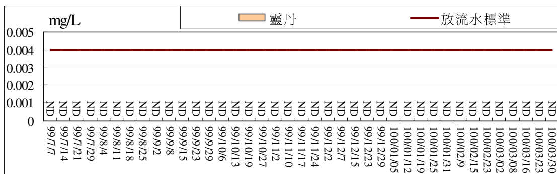
污水處理廠放流口放流水質監測結果比較圖(靈丹)
