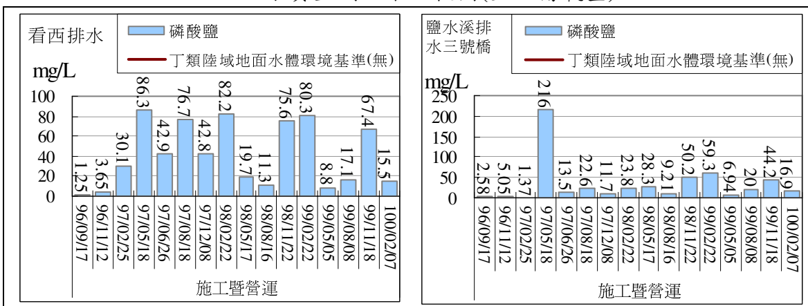
地面水質監測結果比較圖(磷酸鹽)
