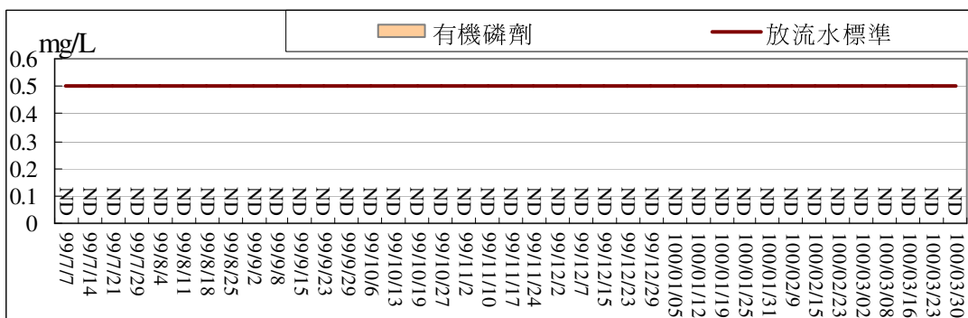
污水處理廠放流口放流水質監測結果比較圖(有機磷劑)
