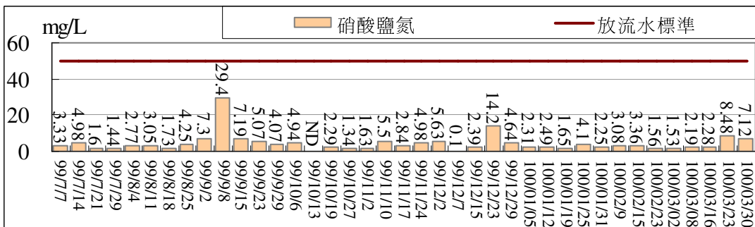
污水處理廠放流口放流水質監測結果比較圖(硝酸鹽氮)
