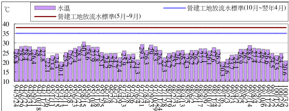
工區放流口放流水質監測結果比較圖(水溫)
