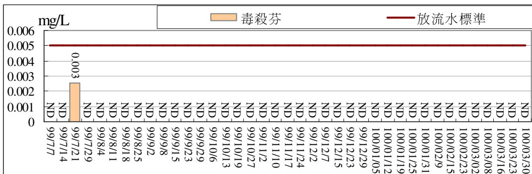
污水處理廠放流口放流水質監測結果比較圖(毒殺芬)
