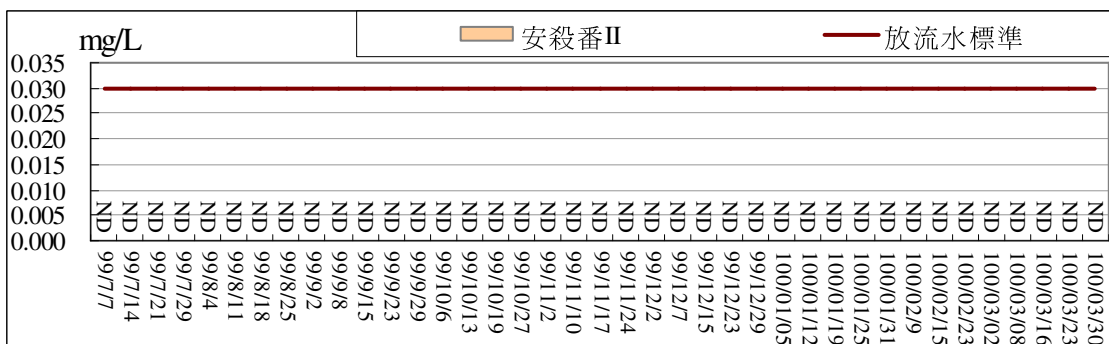
污水處理廠放流口放流水質監測結果比較圖(安殺番 II)
