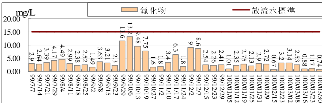
污水處理廠放流口放流水質監測結果比較圖(氟化物)
