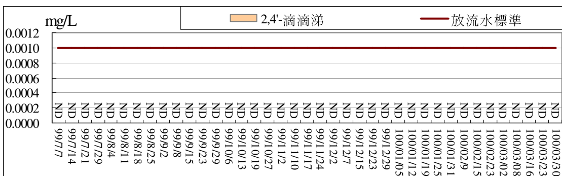
污水處理廠放流口放流水質監測結果比較圖(2,4'-滴滴涕)
