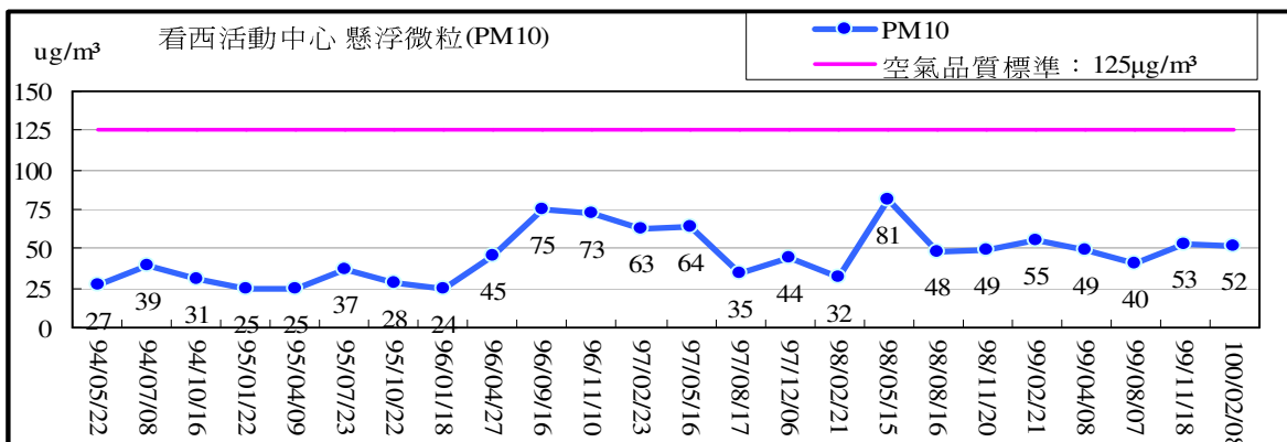
空氣品質監測結果比較圖(看西活動中心 PM10)
