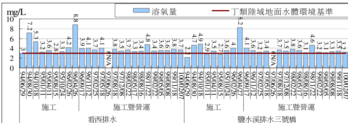
地面水質監測結果比較圖(溶氧量)
