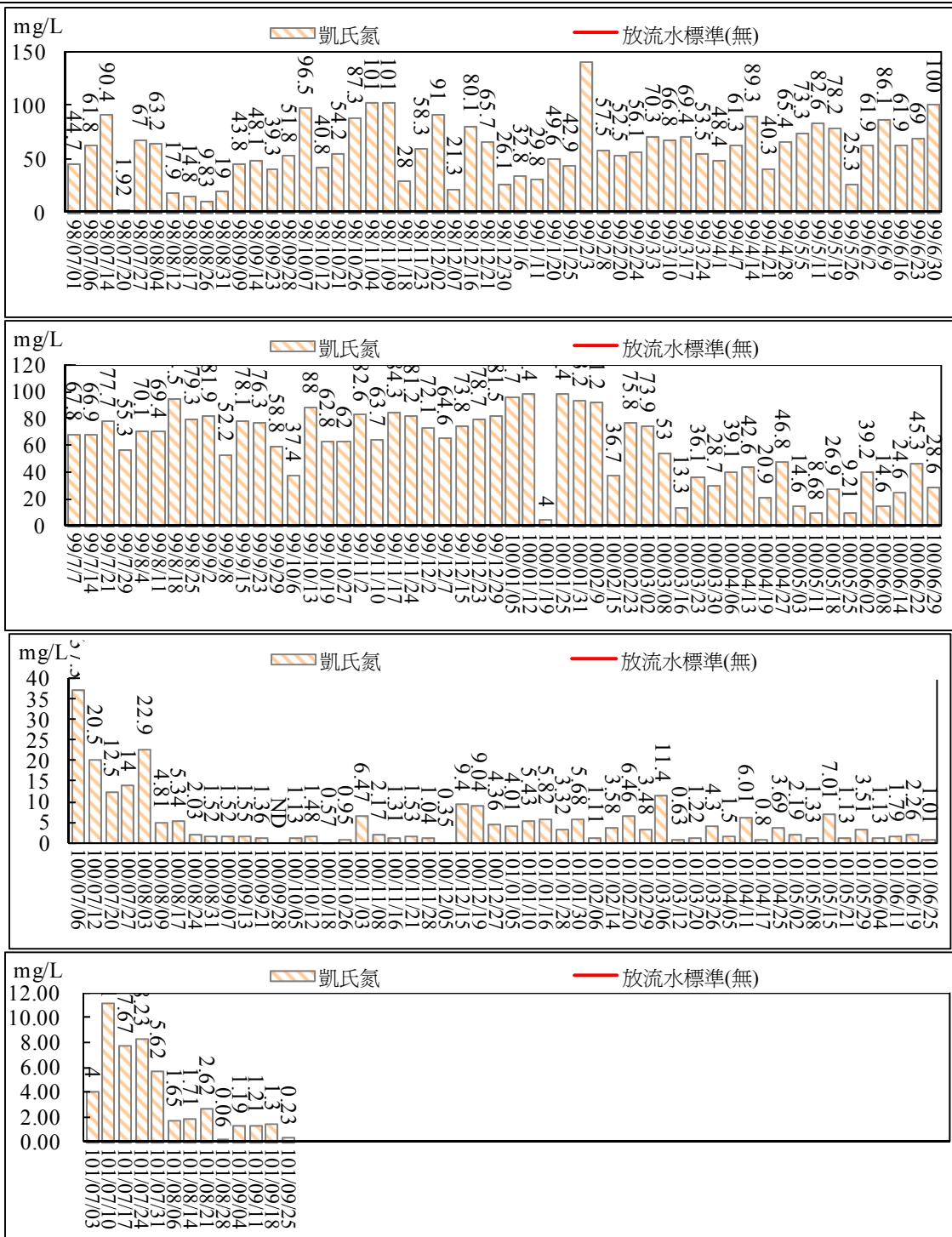
圖 2.28 污水處理廠放流口放流水質監測結果比較圖(凱氏氮)
