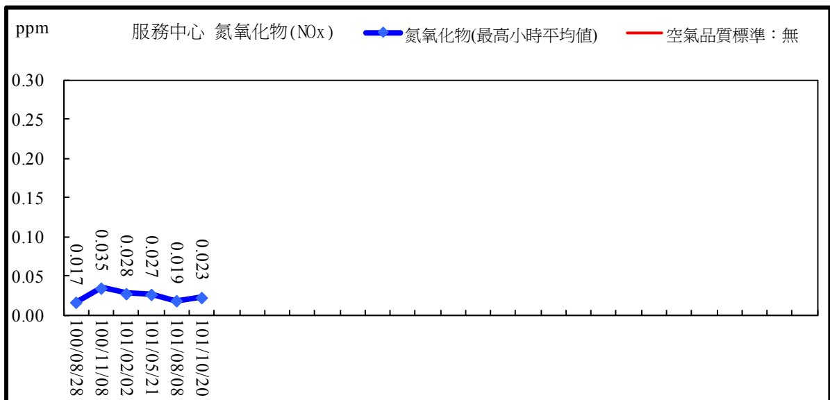
圖 2.14 空氣品質監測結果比較圖(氮氧化物最高小時平均值)
