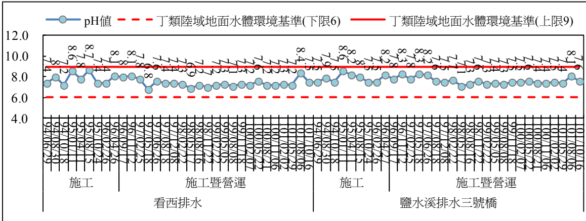
圖 2.69 地面水質監測結果比較圖(pH 值)
