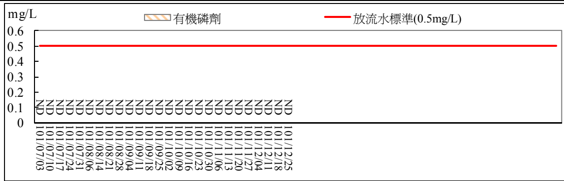
圖 2.60 污水處理廠放流口放流水質監測結果比較圖(有機磷劑)
