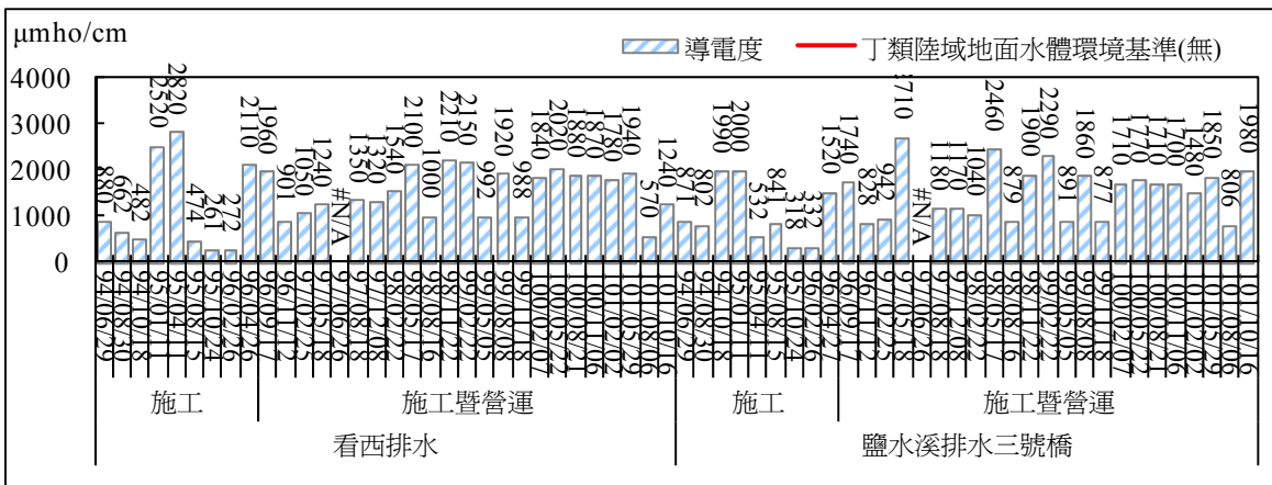
圖 2.70 地面水質監測結果比較圖(導電度)
