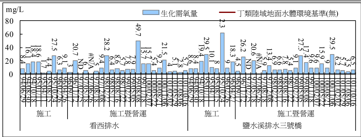
圖 2.61 地面水質監測結果比較圖(生化需氧量)
