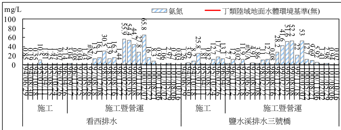
圖 2.64 地面水質監測結果比較圖(氨氮)
