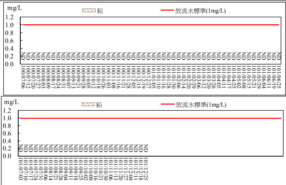
圖 2.41 污水處理廠放流口放流水質監測結果比較圖(鉛)
