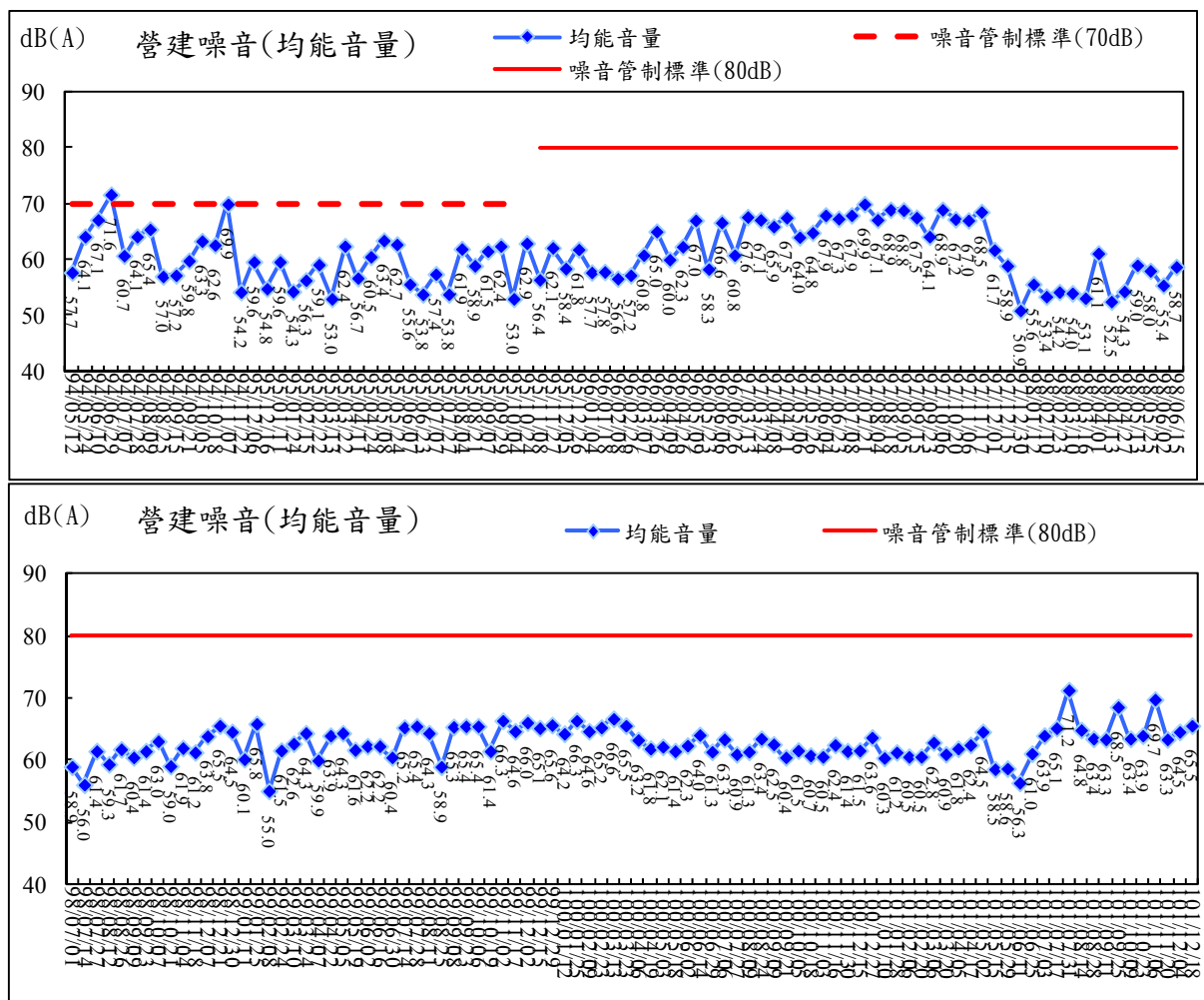
圖 2.79 營建噪音(均能音量)監測結果比較圖
