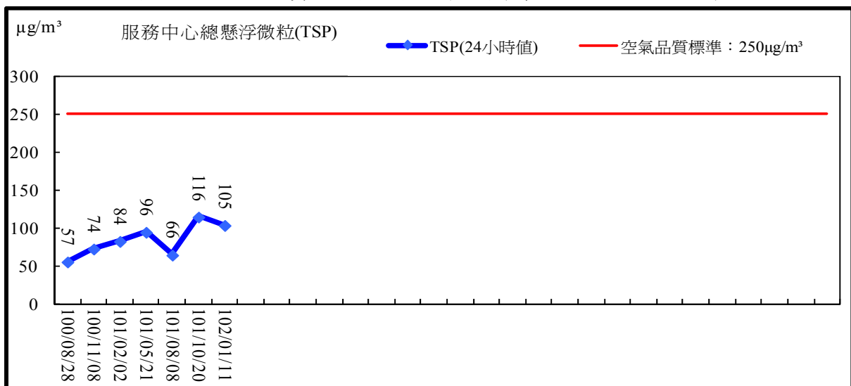
圖 2.3 空氣品質監測結果比較圖 (服務中心 TSP)
