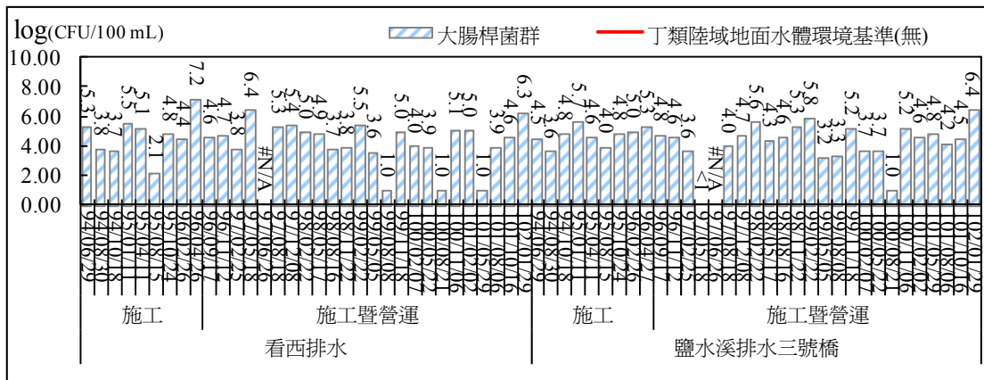
圖 2.67 地面水質監測結果比較圖(大腸桿菌群)
