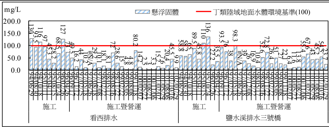
圖 2.65 地面水質監測結果比較圖(懸浮固體)
