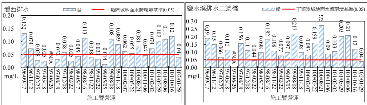
圖 2.63 地面水質監測結果比較圖(錳)
