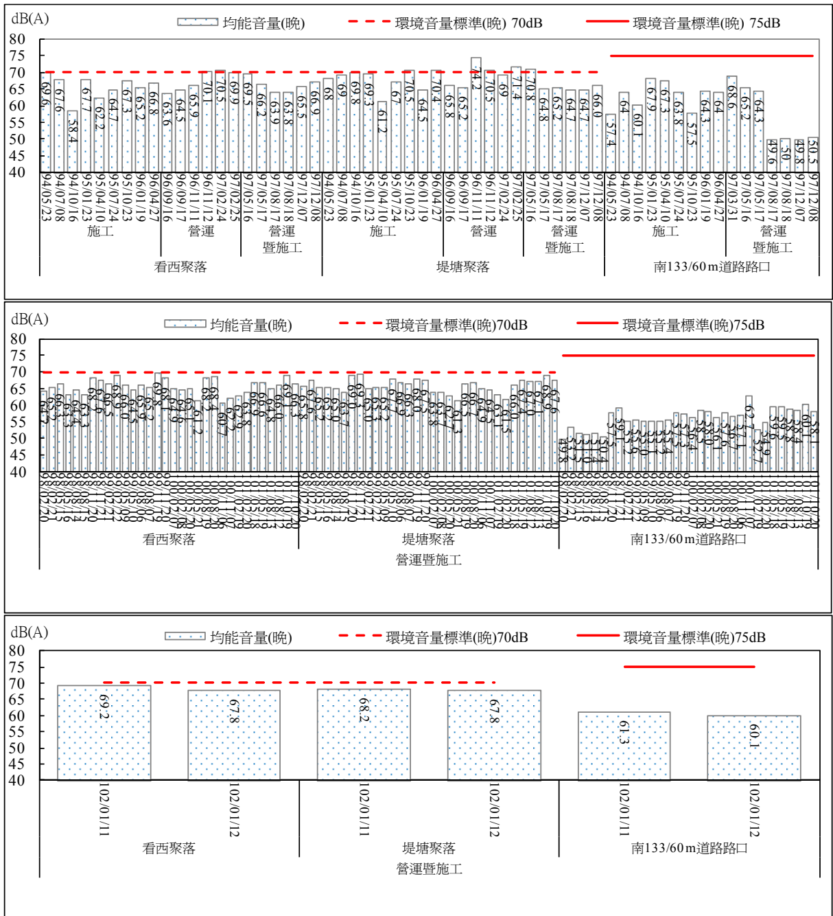
圖 2.75 環境噪音監測結果比較圖(晚間)
