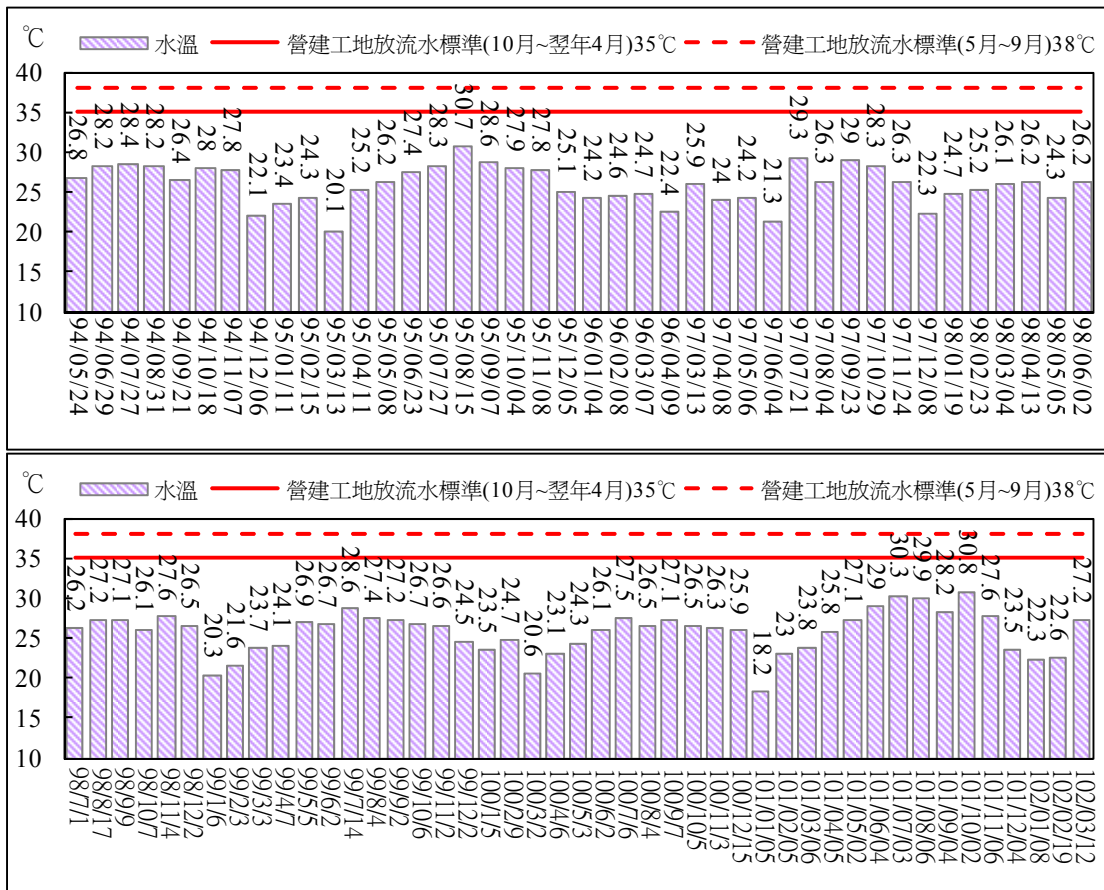
圖 2.86 工區放流口放流水質監測結果比較圖(水溫)
