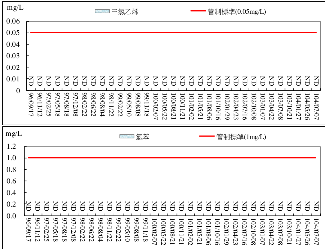
圖 2.72 地下水水質監測結果比較圖
