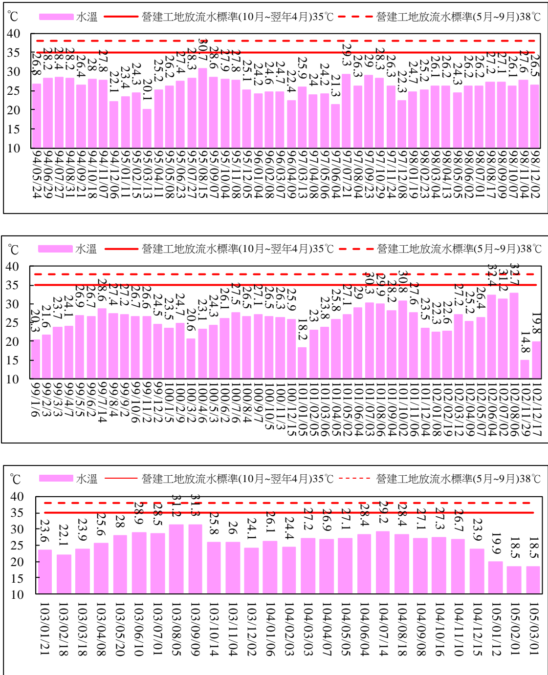
圖 2.86 工區放流口放流水質監測結果比較圖(水溫)
