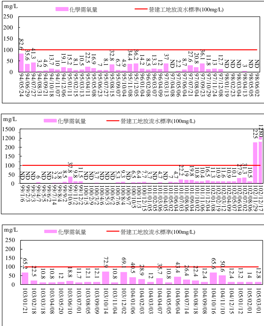
圖 2.82 工區放流口放流水質監測結果比較圖(化學需氧量)
