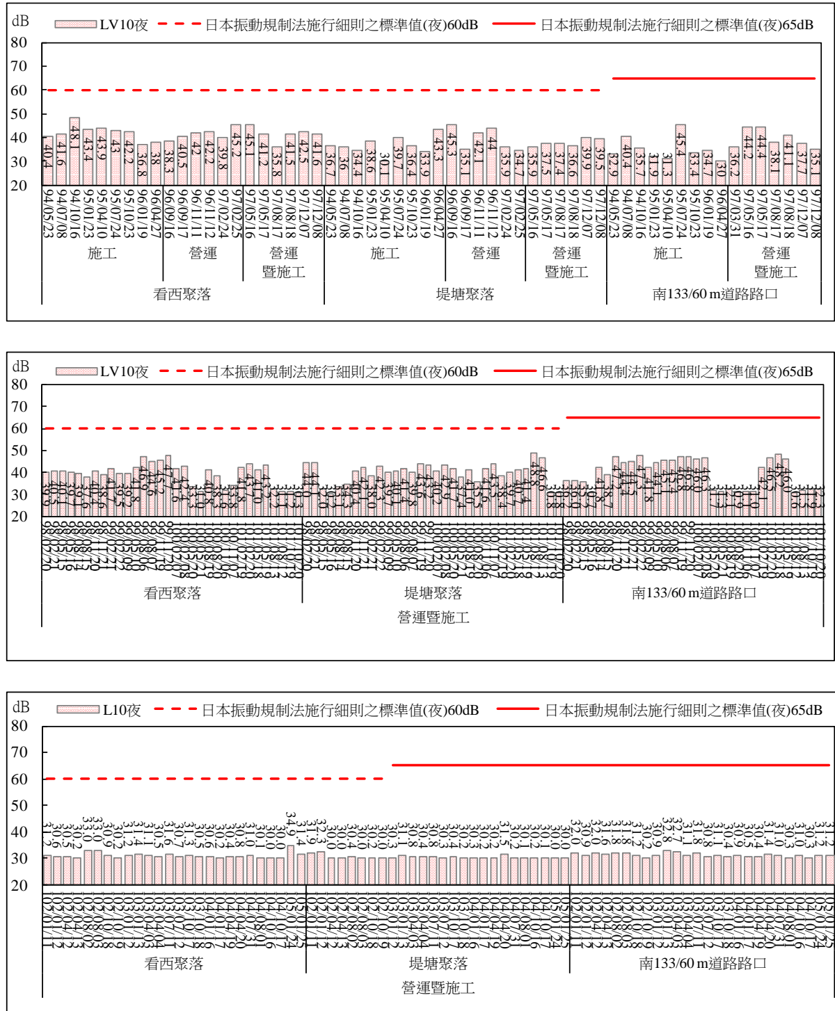
圖 2.78 環境振動監測結果比較圖(夜間)
