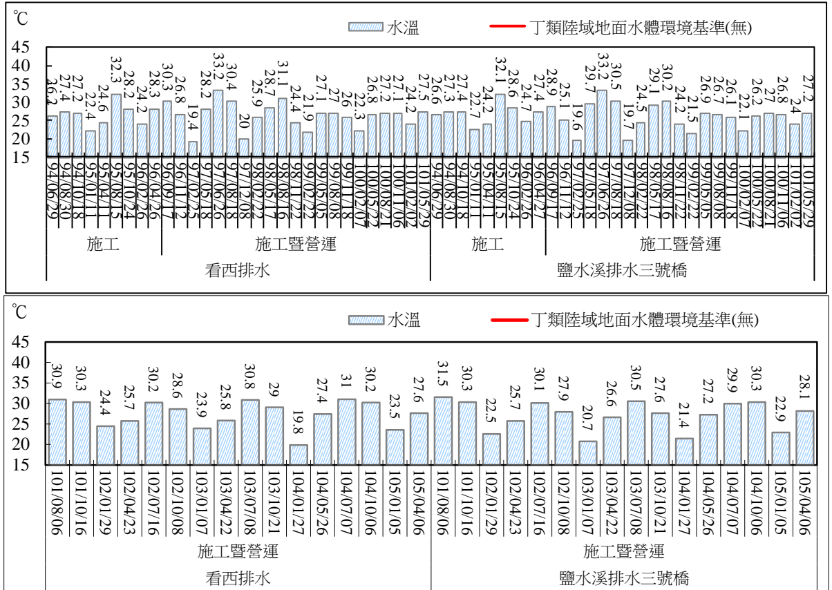
圖 2.68 地面水質監測結果比較圖(水溫)
