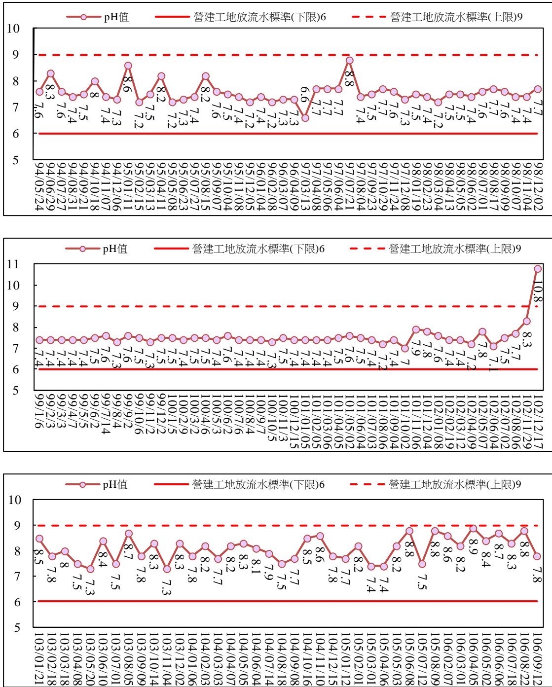
圖 2.87 工區放流口放流水質監測結果比較圖(pH 值)
