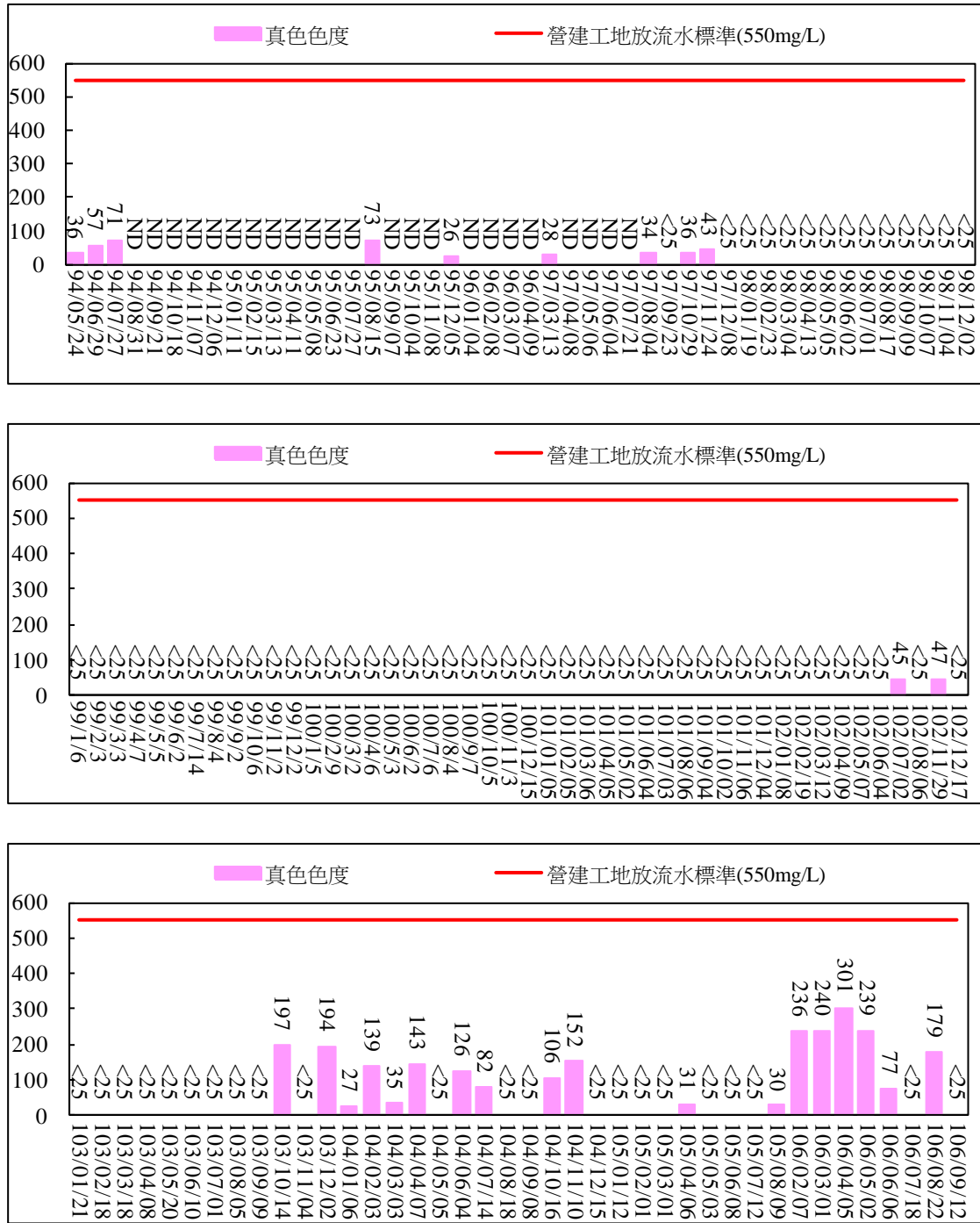
圖 2.85 工區放流口放流水質監測結果比較圖(真色色度)
