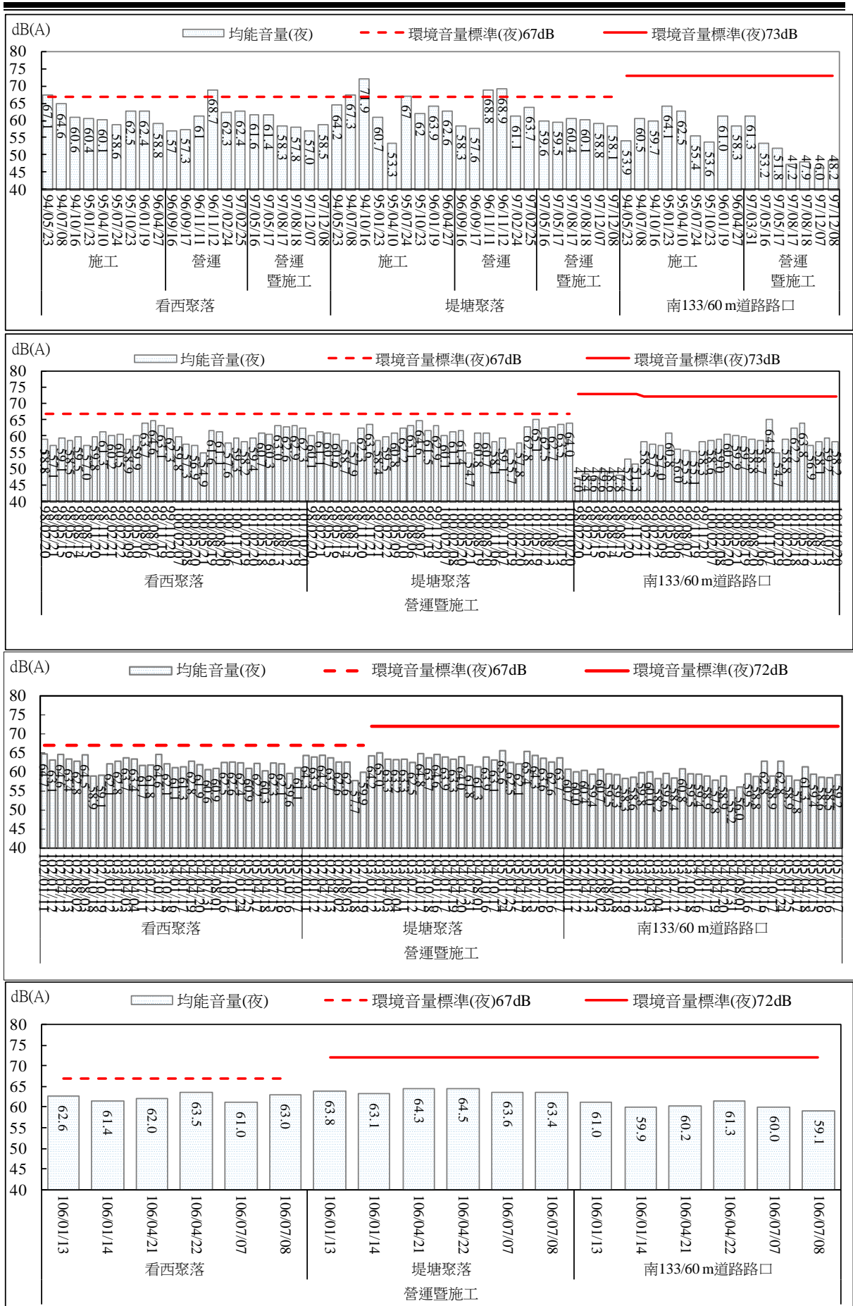
圖 2.76 環境噪音監測結果比較圖(夜間)
