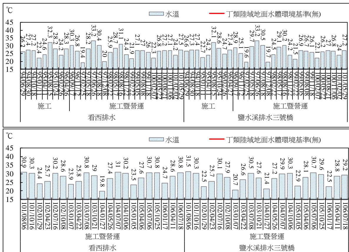
圖 2.68 地面水質監測結果比較圖(水溫)
