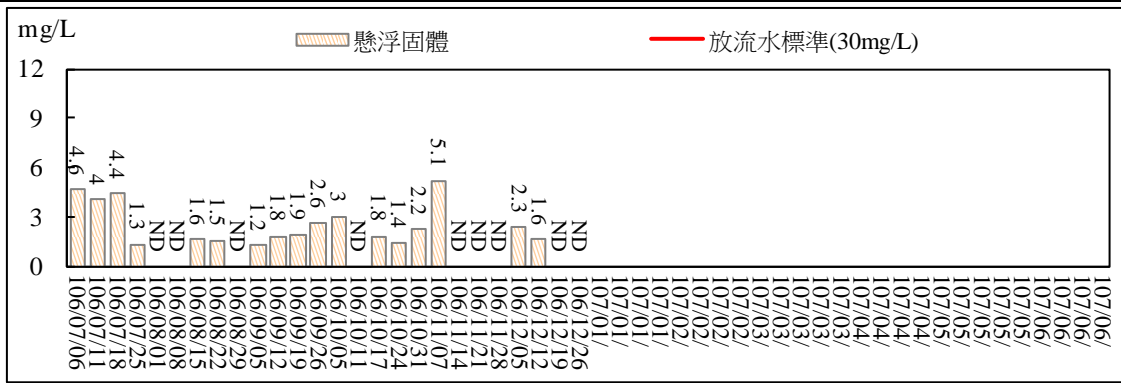
圖 2.30 污水處理廠放流口放流水質監測結果比較圖(懸浮固體)
