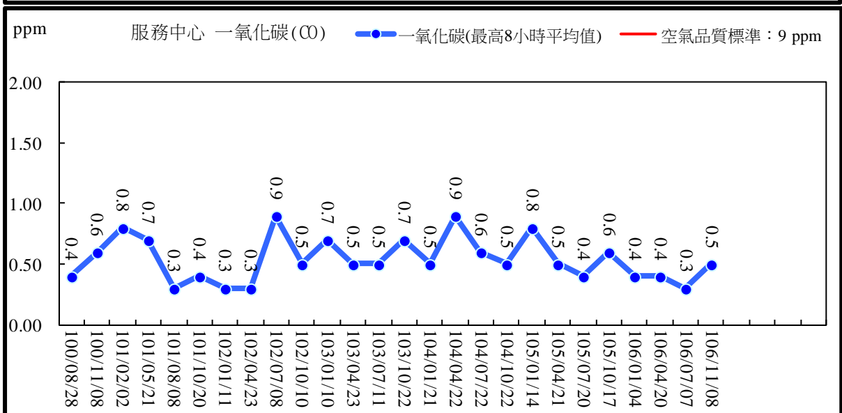
圖 2.15 空氣品質監測結果比較圖(一氧化碳最高八小時平均值)
