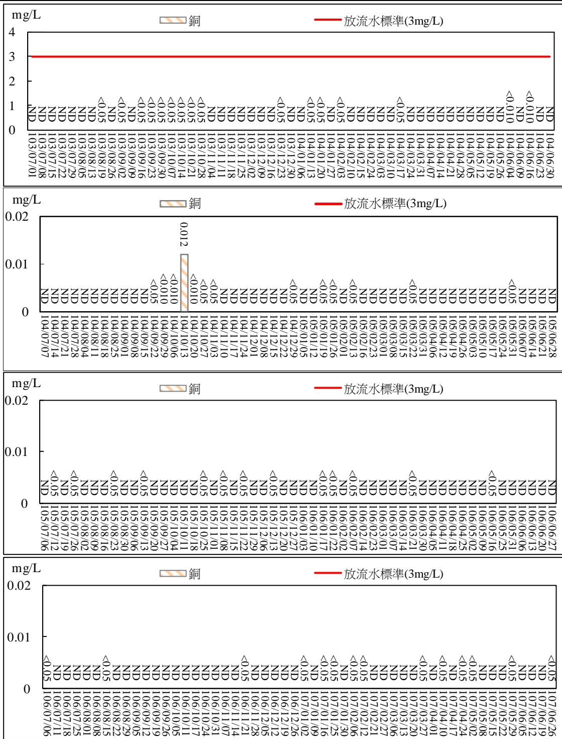
圖 2.43 污水處理廠放流口放流水質監測結果比較圖(銅)
