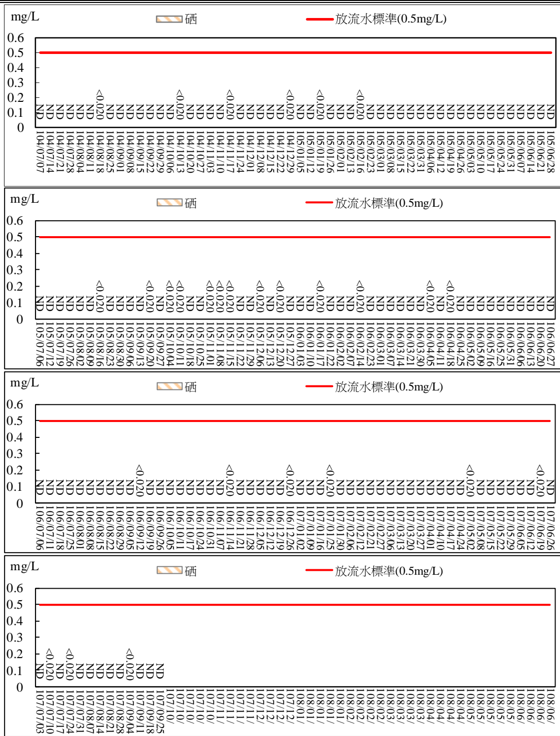
圖 2.46 污水處理廠放流口放流水質監測結果比較圖(硒)
