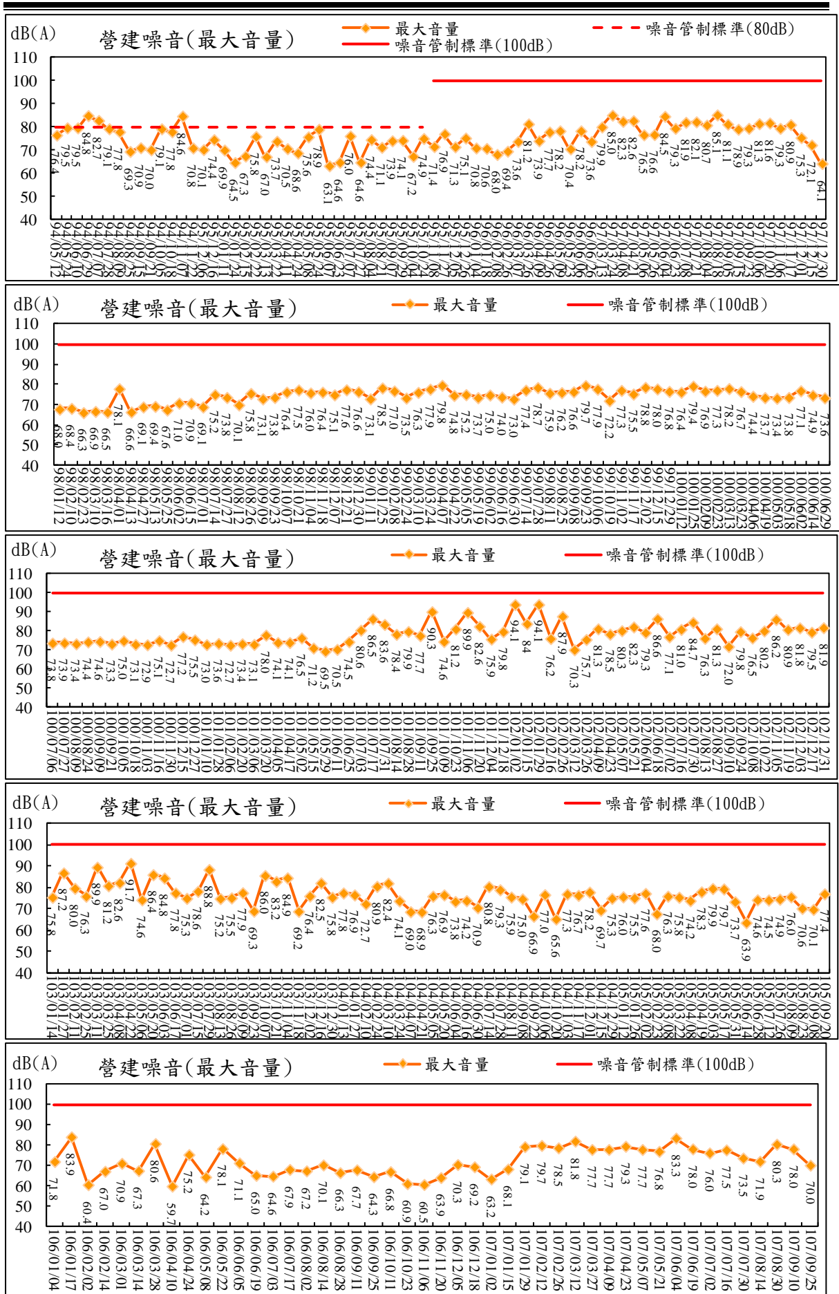
圖 2.80 營建噪音(最大音量)監測結果比較圖
