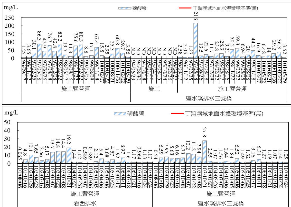
圖 2.62 地面水質監測結果比較圖(磷酸鹽)
