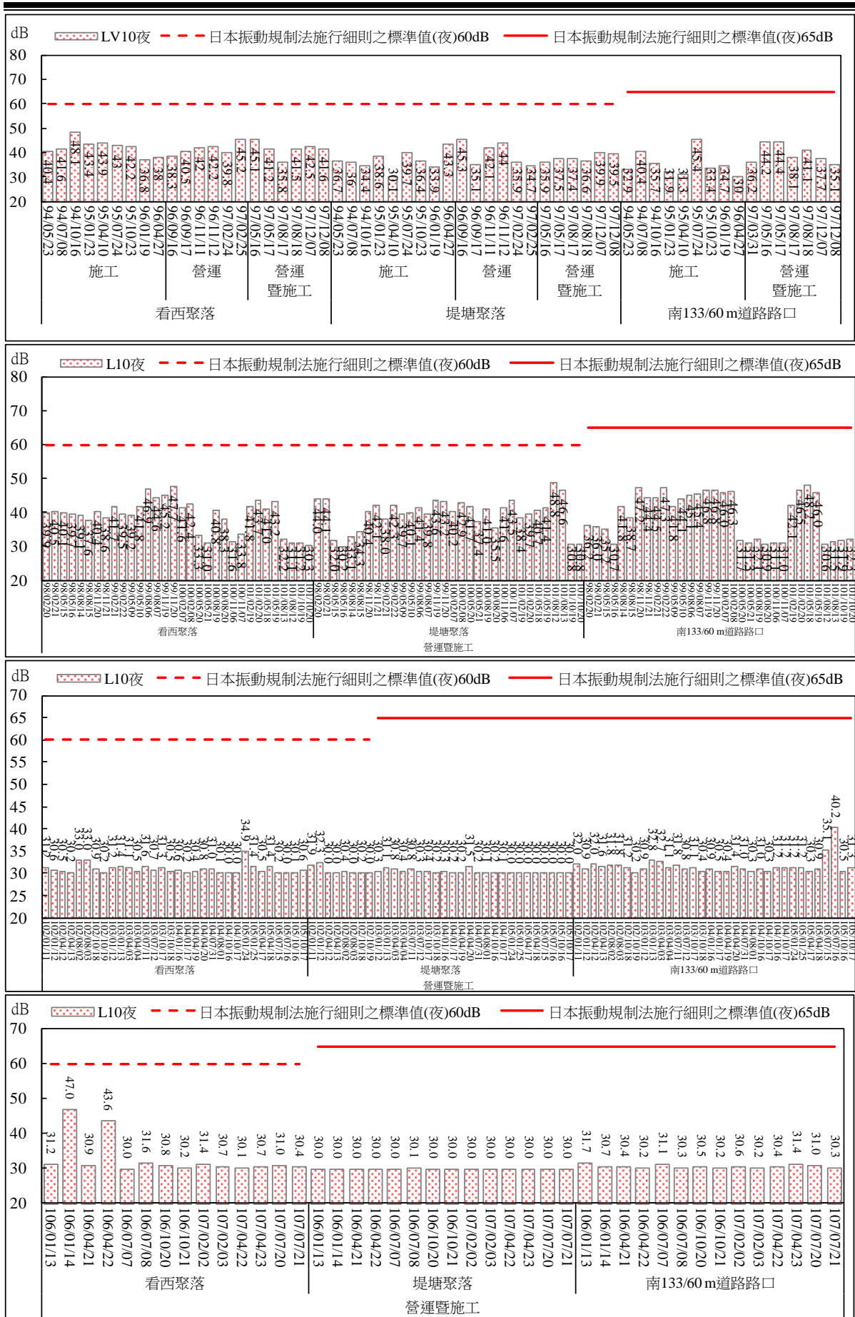
圖 2.78 環境振動監測結果比較圖(夜間)
