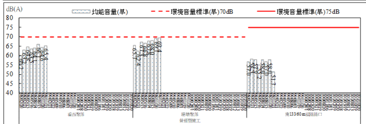
圖 2.73 環境噪音監測結果比較圖(早間)
