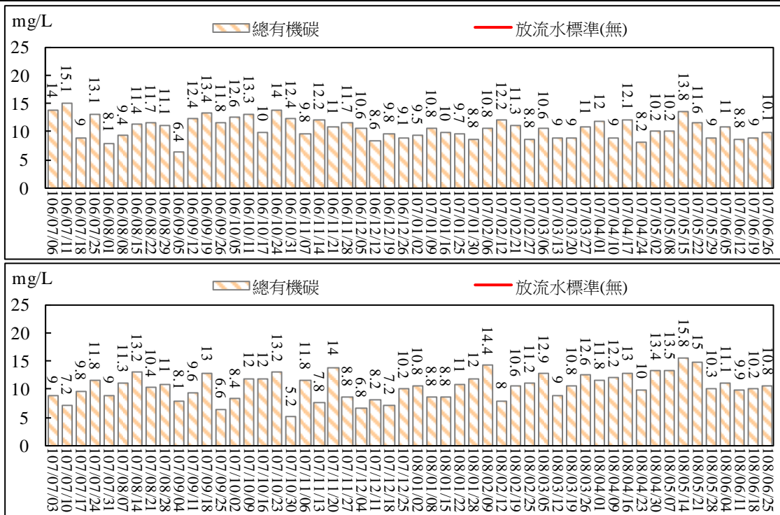
圖 2.34 污水處理廠放流口放流水質監測結果比較圖(總有機碳)
