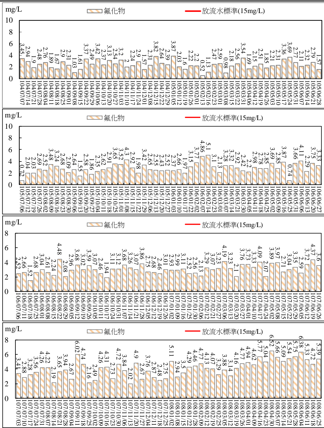
圖 2.35 污水處理廠放流口放流水質監測結果比較圖(氟化物)
