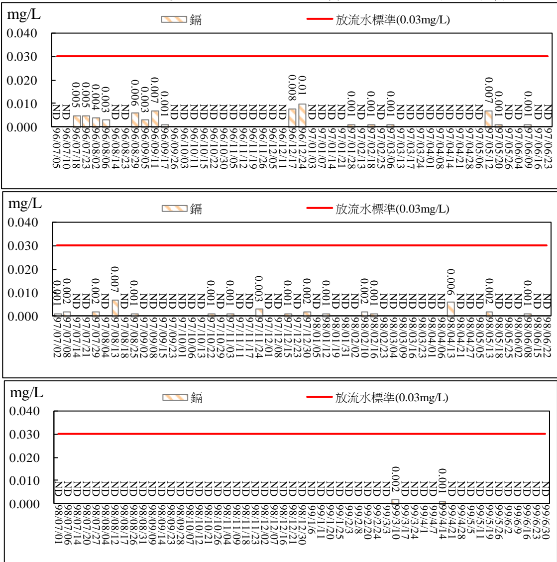
圖 2.39 污水處理廠放流口放流水質監測結果比較圖(鎘)
