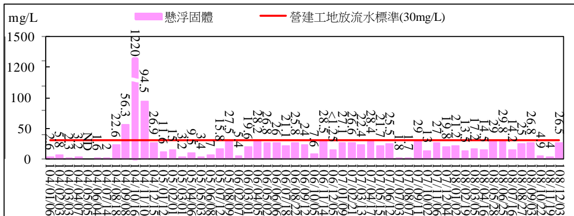
圖 2.83 工區放流口放流水質監測結果比較圖(懸浮固體)
