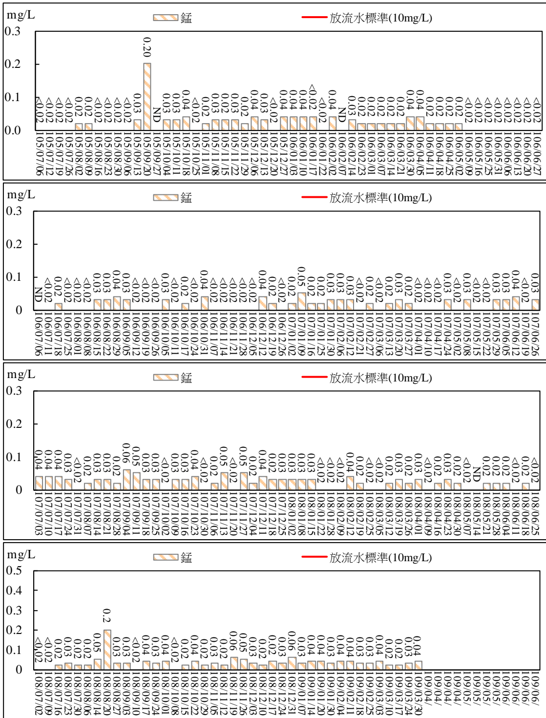
圖 2.42 污水處理廠放流口放流水質監測結果比較圖(錳)
