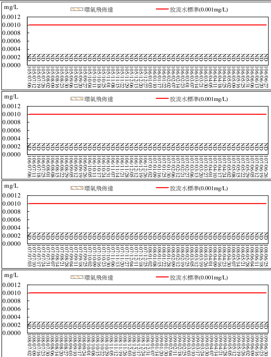
圖 2.52 污水處理廠放流口放流水質監測結果比較圖(環氧飛佈達)
