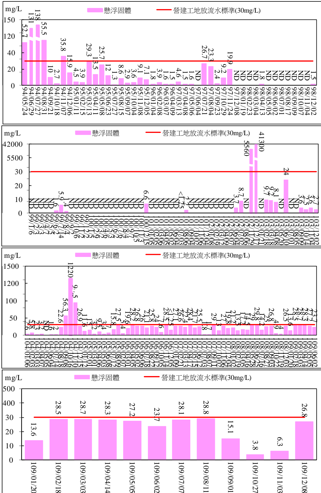
圖 2.83 工區放流口放流水質監測結果比較圖(懸浮固體)
