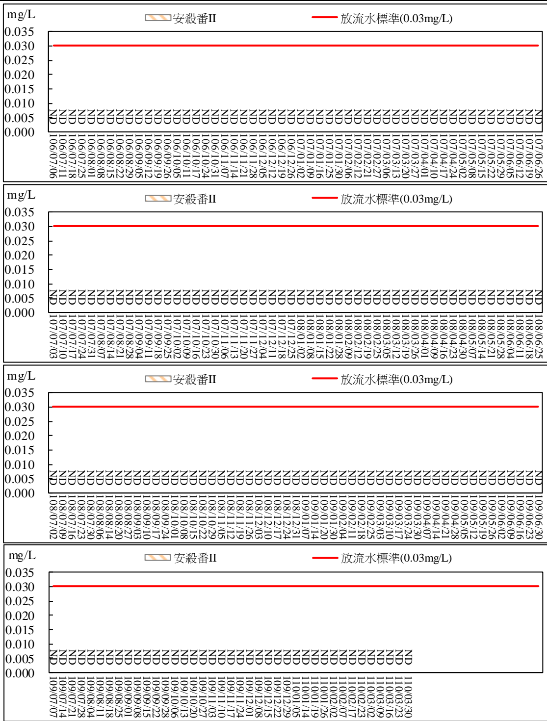
圖 2.50 污水處理廠放流口放流水質監測結果比較圖(安殺番 II)
