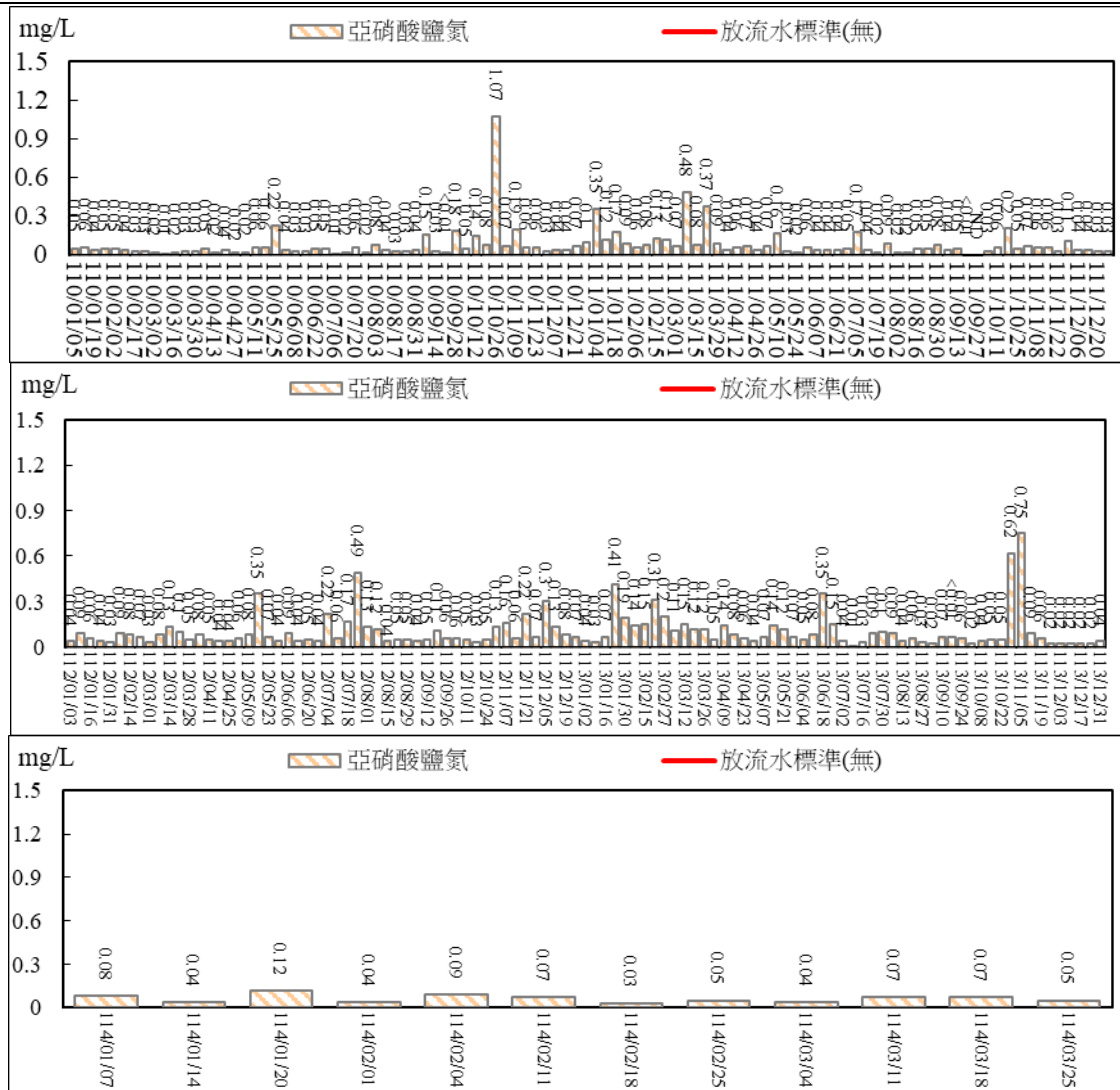
圖 2.24 污水處理廠放流口放流水質監測結果比較圖(亞硝酸鹽氮)
