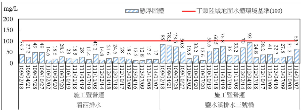
圖 2.60 地面水質監測結果比較圖(懸浮固體)
