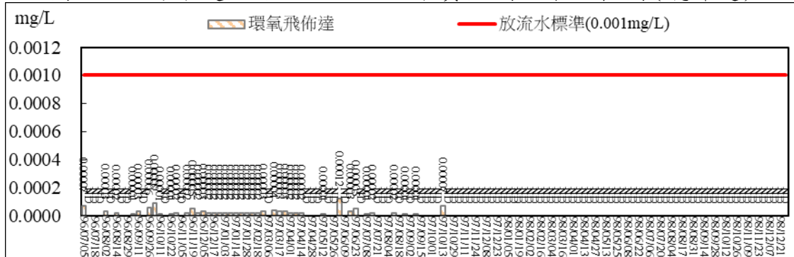
圖 2.48 污水處理廠放流口放流水質監測結果比較圖(飛佈達)
