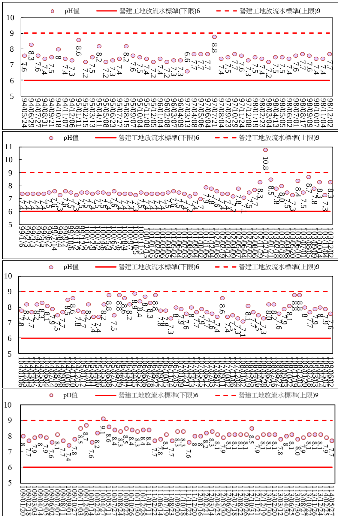
圖 2.85 工區放流口放流水質監測結果比較圖(pH 值)
