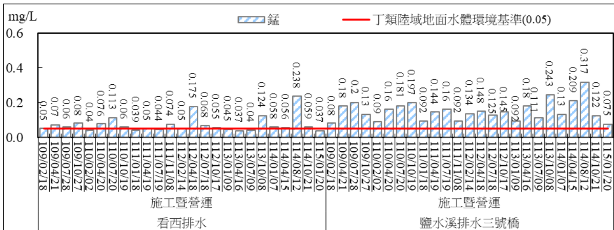
圖 2.69 地面水質監測結果比較圖(錳)
