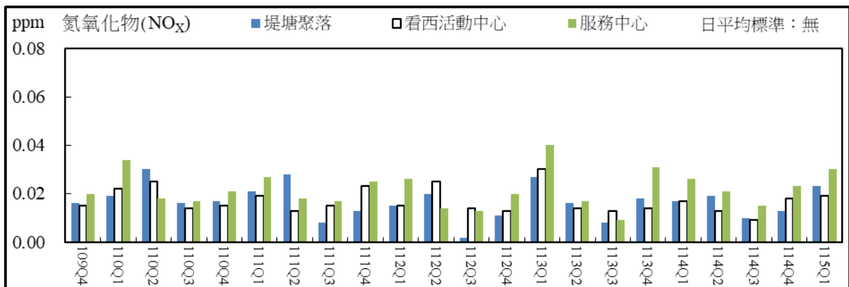
圖 2.10 空氣品質監測結果比較圖(氮氧化物日平均值)
