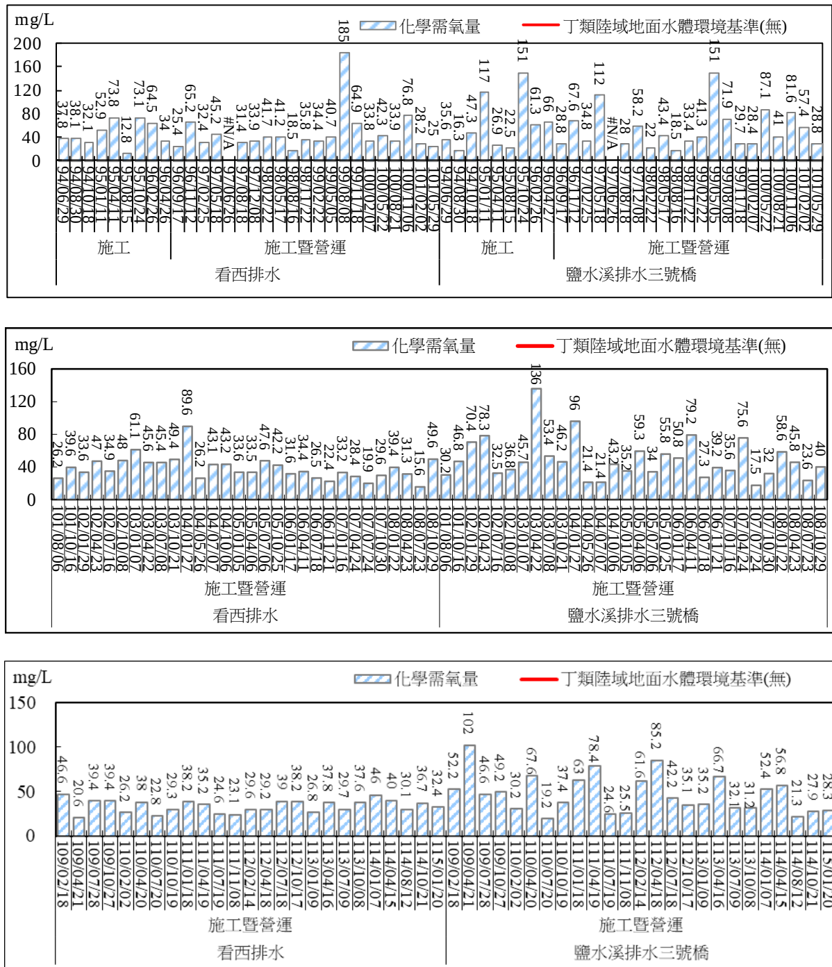
圖 2.63 地面水質監測結果比較圖(化學需氧量)
