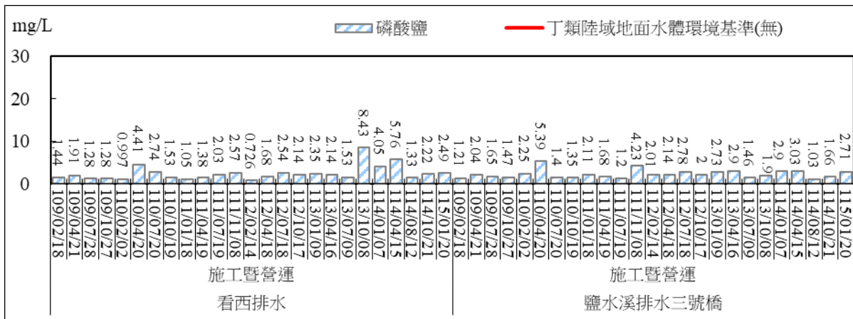
圖 2.60 地面水質監測結果比較圖(磷酸鹽)
