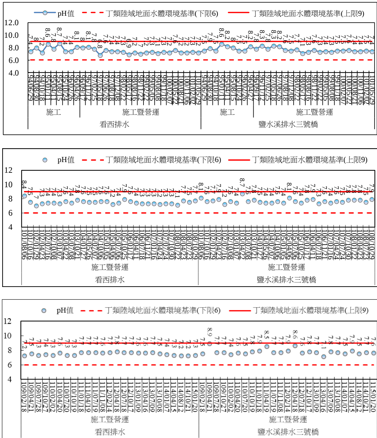
圖 2.66 地面水質監測結果比較圖(pH 值)
