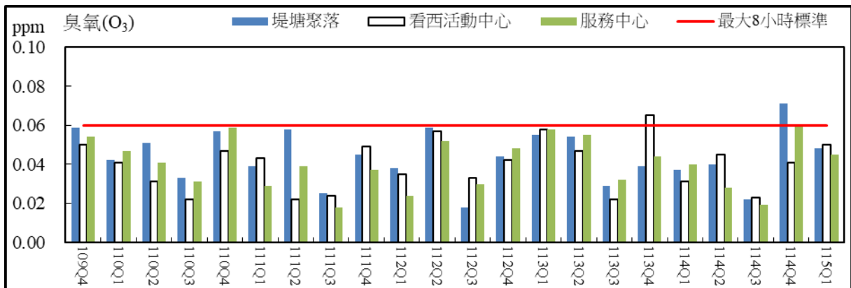
圖 2.14 空氣品質監測結果比較圖(臭氧最大八小時平均值)
