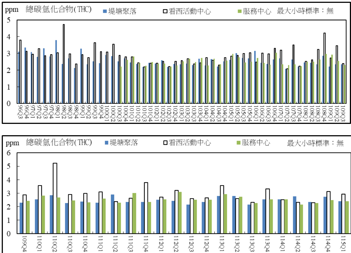
圖 2.21 空氣品質監測結果比較圖(總碳氫化合物最大小時平均值)
