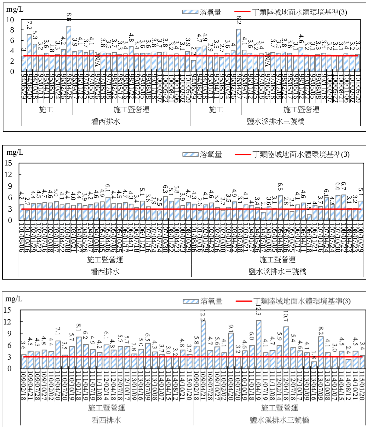
圖 2.68 地面水質監測結果比較圖(溶氧量)
