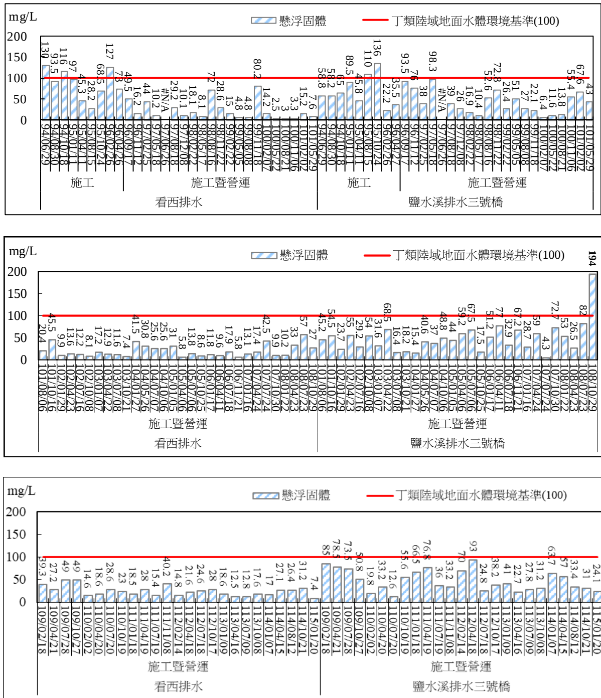
圖 2.61 地面水質監測結果比較圖(懸浮固體)
