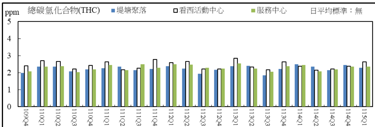
圖 2.20 空氣品質監測結果比較圖(總碳氫化合物日平均值)
