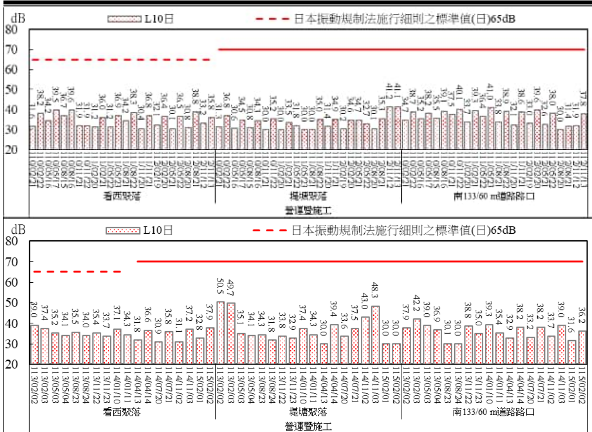
圖 2.75 環境振動監測結果比較圖(日間)
