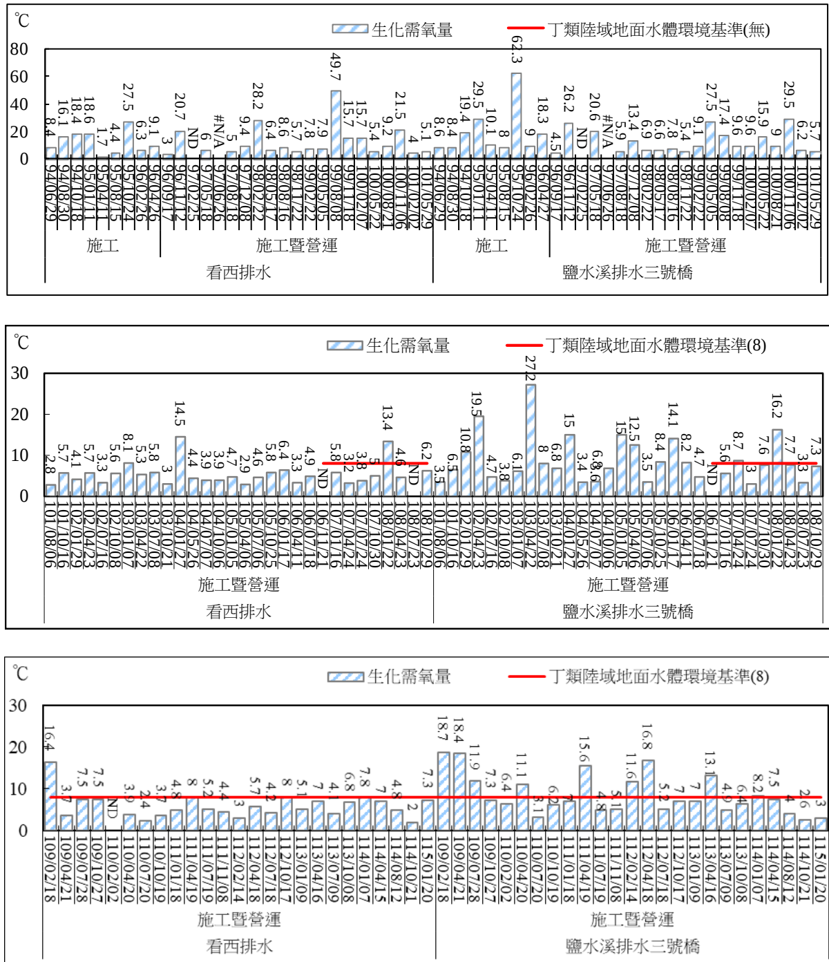
圖 2.59 地面水質監測結果比較圖(生化需氧量)
