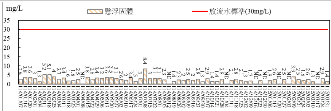
圖 2.27 污水處理廠放流口放流水質監測果比較圖(懸浮固體)
