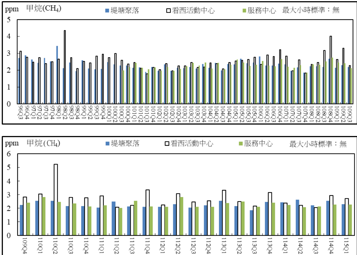
圖 2.17 空氣品質監測結果比較圖(甲烷最大小時平均值)
