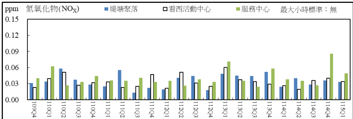
圖 2.11 空氣品質監測結果比較圖(氮氧化物最大小時平均值)
