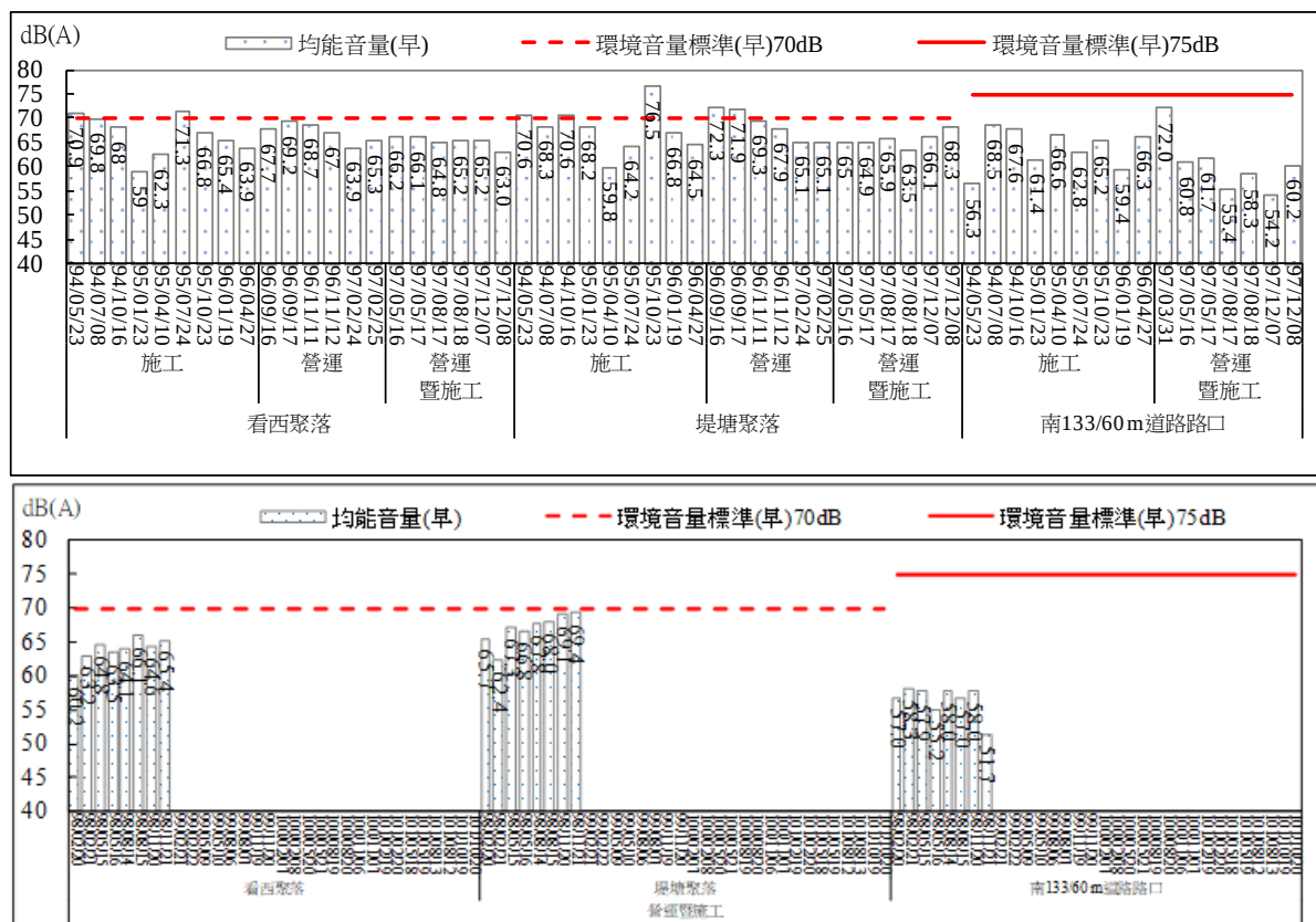
圖 2.71 環境噪音監測結果比較圖(早間)
