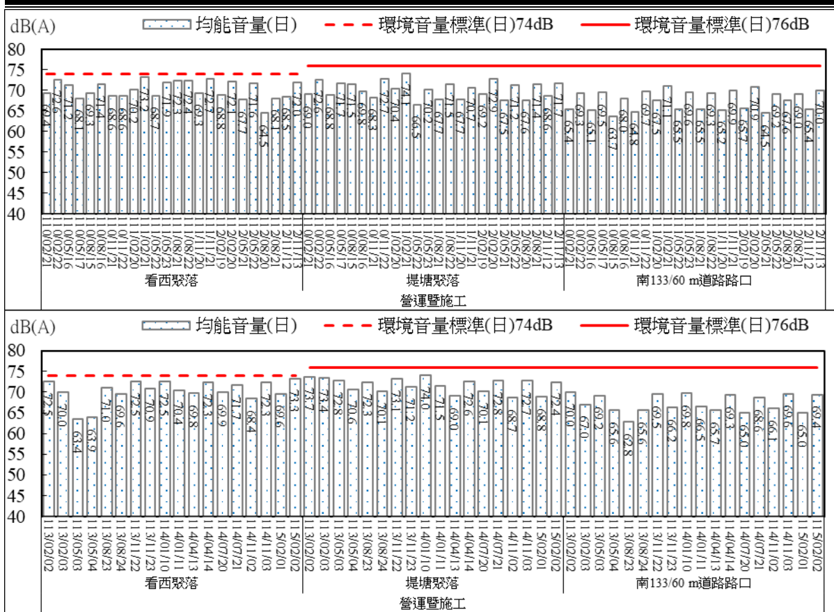
圖 2.72 環境噪音監測結果比較圖(日間)
