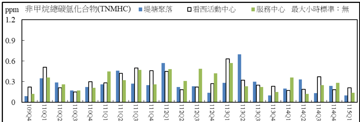
圖 2.19 空氣品質監測結果比較圖(非甲烷總碳氫化合物最大小時平均值)
