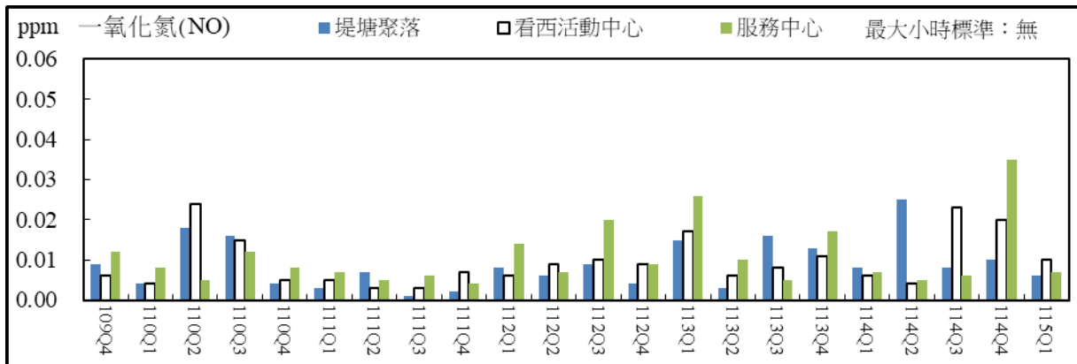
圖 2.9 空氣品質監測結果比較圖(一氧化氮最大小時平均值)
