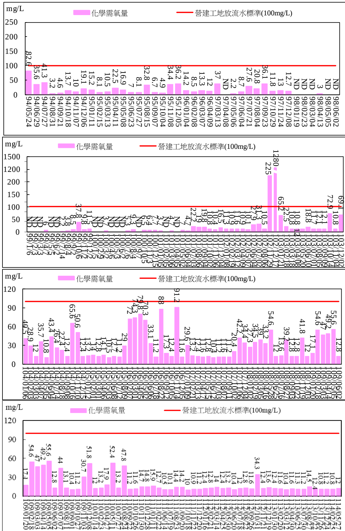
圖 2.80 工區放流口放流水質監測結果比較圖(化學需氧量)
