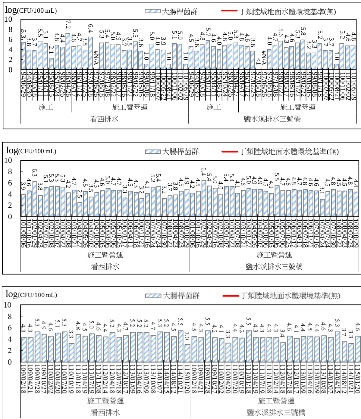
圖 2.64 地面水質監測結果比較圖(大腸桿菌群)
