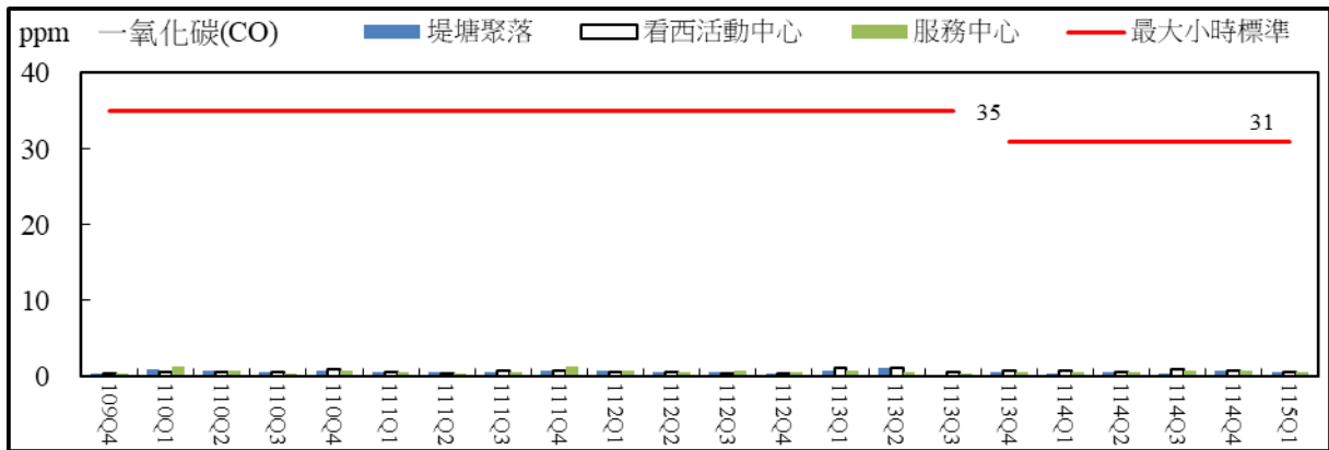
圖 2.13 空氣品質監測結果比較圖(一氧化碳最大小時平均值)
