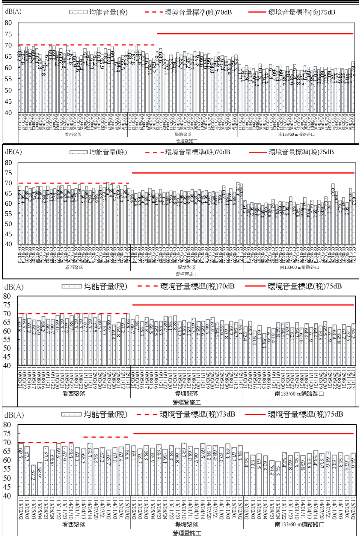
圖 2.73 環境噪音監測結果比較圖(晚間)
