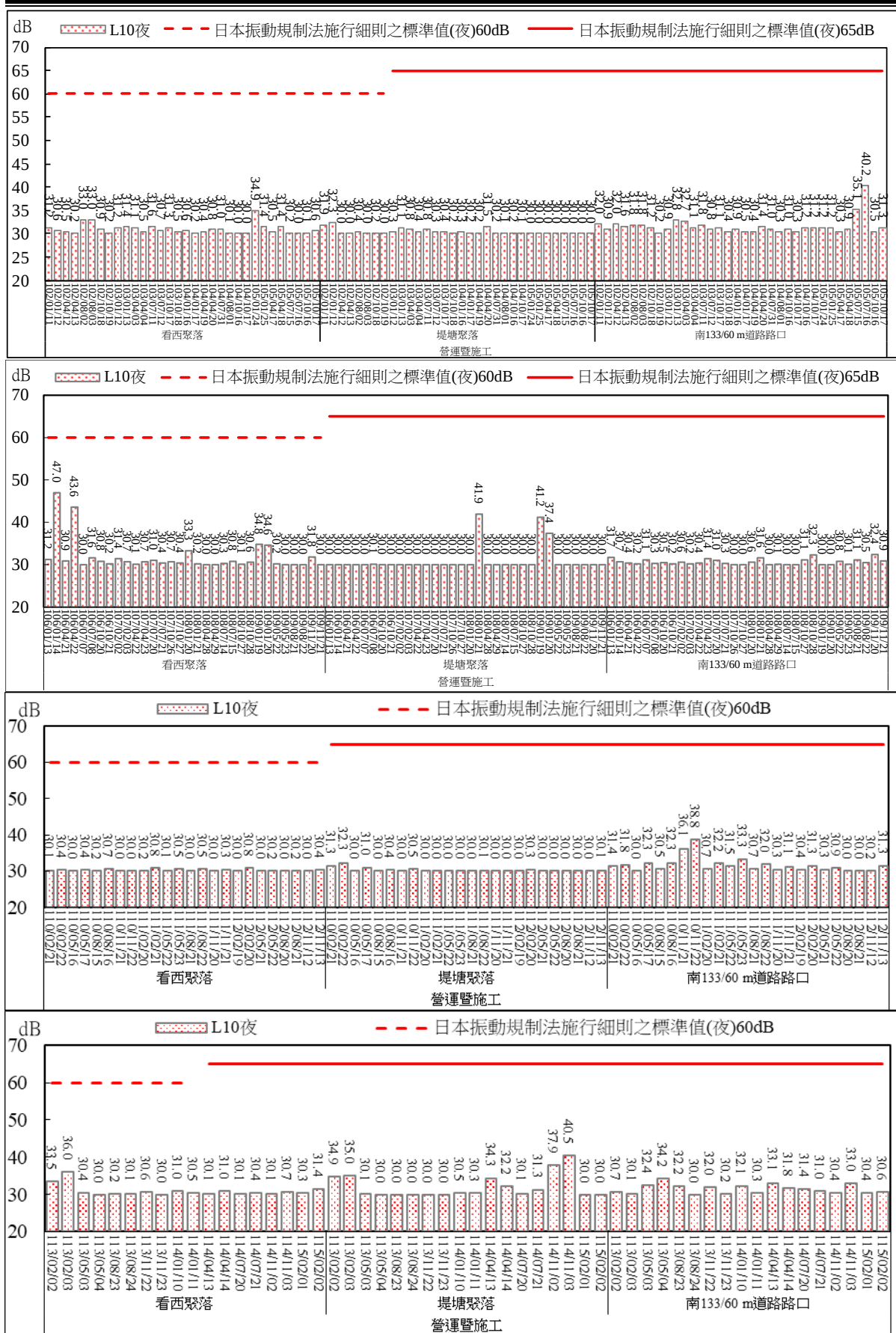
圖 2.76 環境振動監測結果比較圖(夜間)
