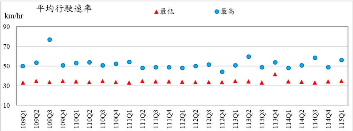
圖 2.86 交通量平均行駛速率監測結果圖
