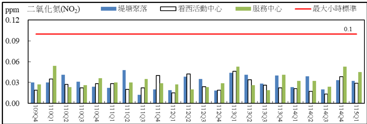
圖 2.7 空氣品質監測結果比較圖(二氧化氮最大小時平均值)
