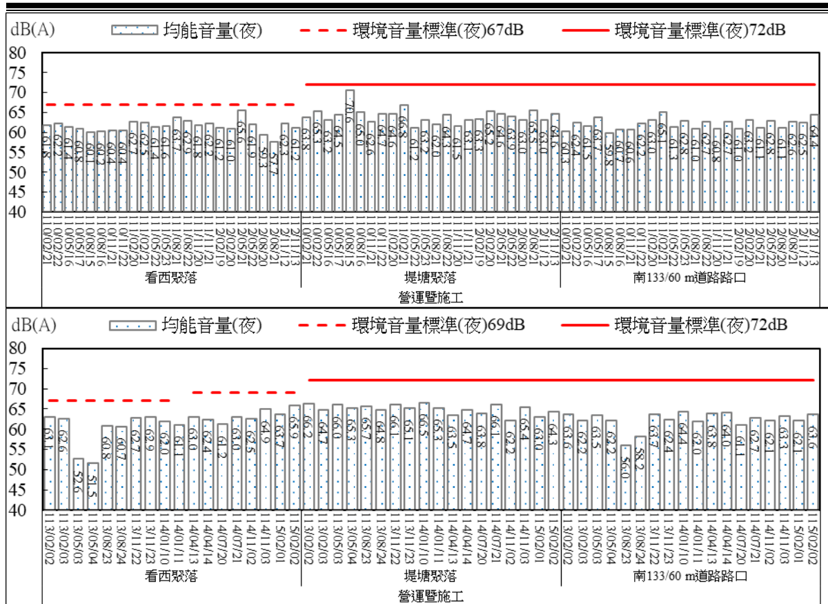
圖 2.74 環境噪音監測結果比較圖(夜間)
