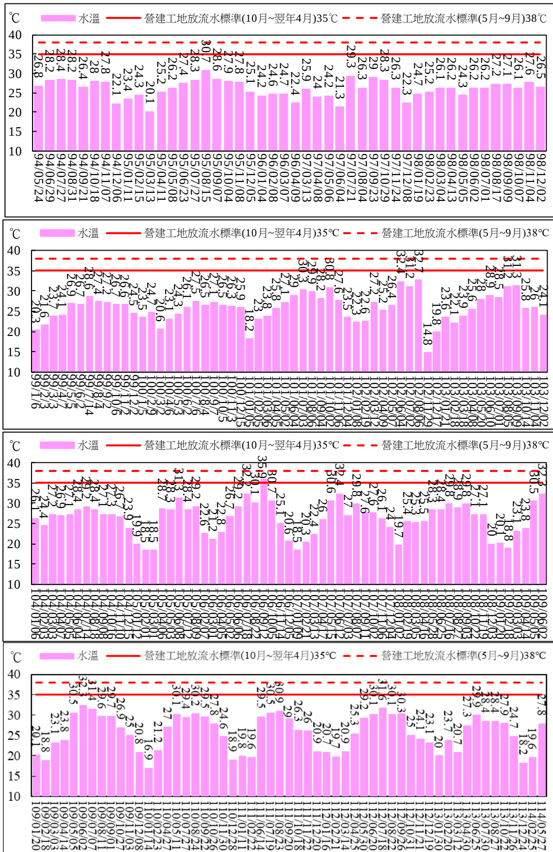
圖 2.84 工區放流口放流水質監測結果比較圖(水溫)
