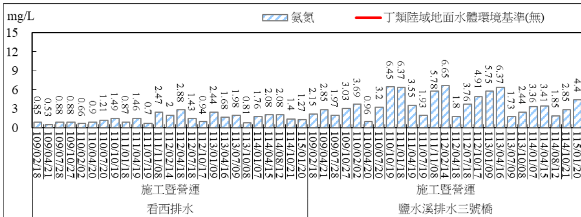
圖 2.62 地面水質監測結果比較圖(氨氮)
