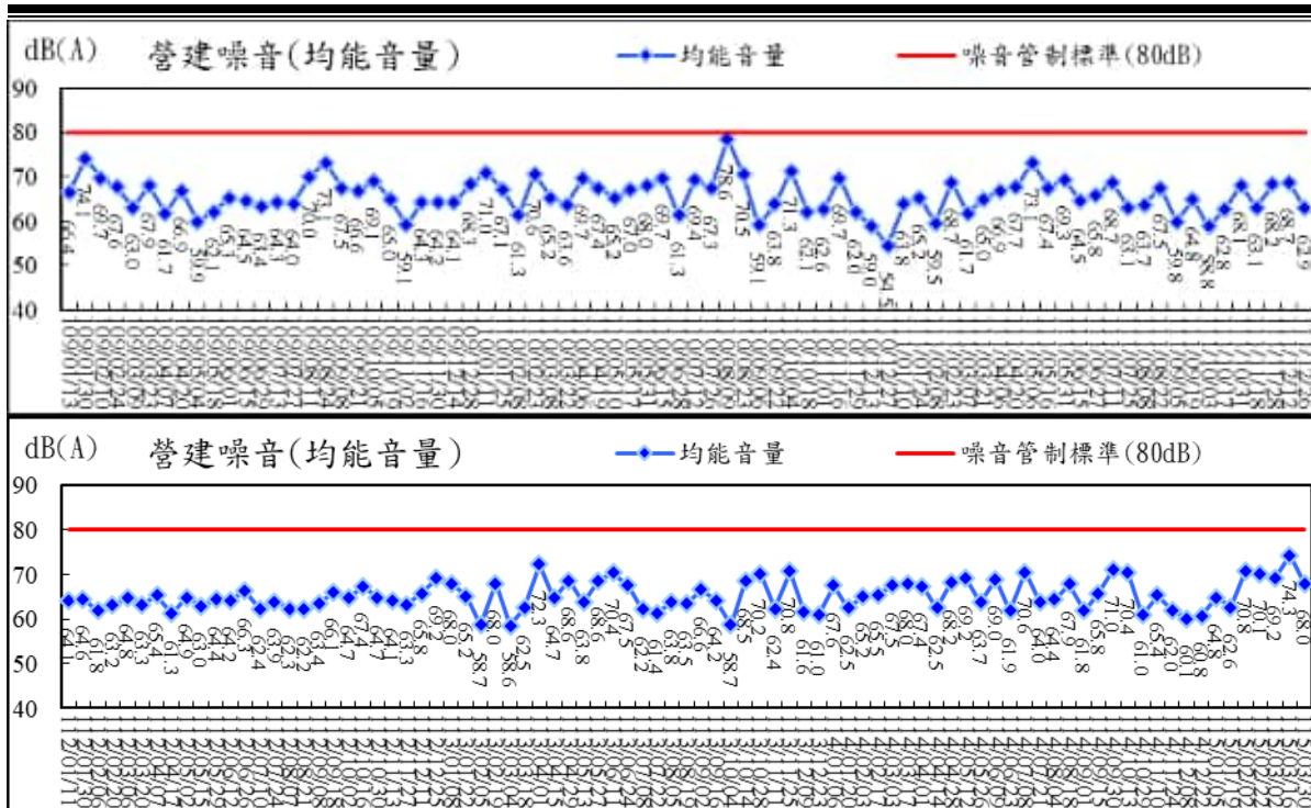
圖 2.77 營建噪音(均能音量)監測結果比較圖
