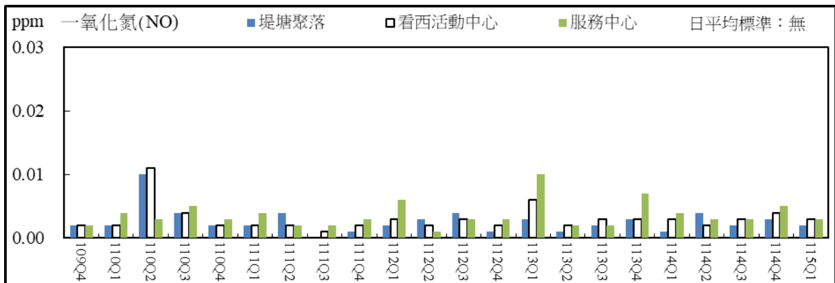
圖 2.8 空氣品質監測結果比較圖(一氧化氮日平均值)
