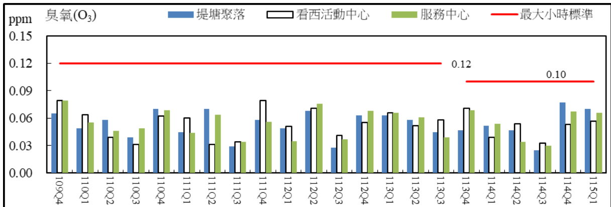
圖 2.15 空氣品質監測結果比較圖(臭氧最大小時平均值)
